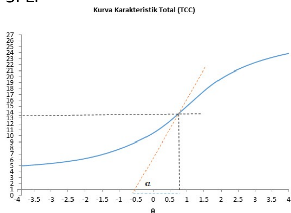
Gambar 2. Kurva karakteristik total model 3PL
